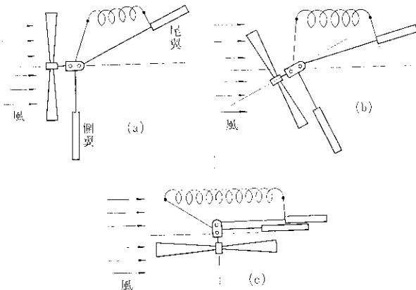
第 2 図 偏向装置による制御
