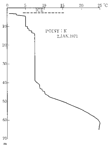
観測点 K での温度分布 (1971.1.2)
