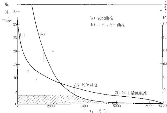
第 6 図 風況曲線とエネルギー曲線 (昭和基地 1961 年)
