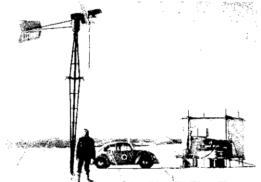
第 1 図 モーション基地の風力発電機（翼径 3 m）
