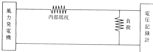
図-6 昭和基地における結線図
