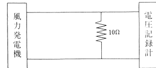
(b) 電力測定用 負荷直結回路
