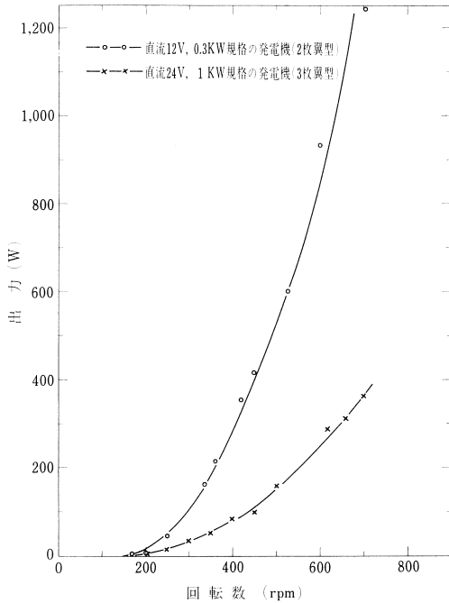
図-2 使用発電機の回転数と出力の関係
