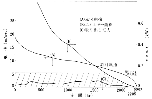
図—10 (b) 内陸基地における風況曲線とエネルギー曲線
