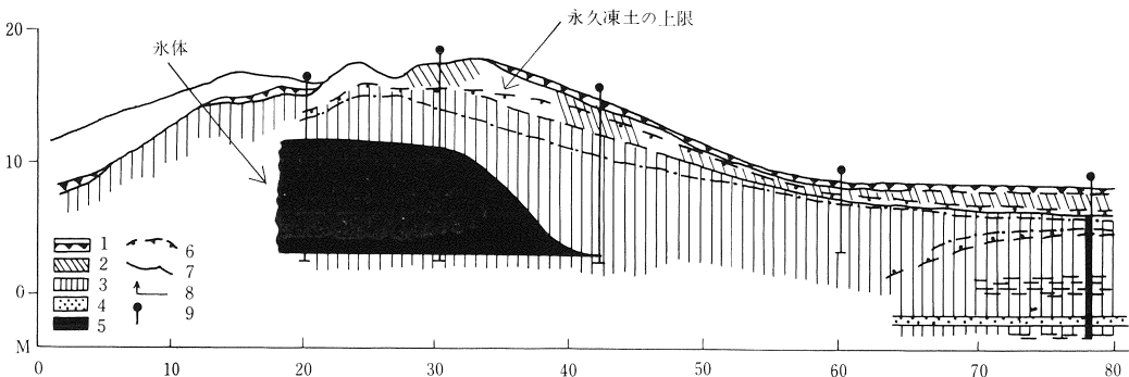
図—3 ピンゴ（図—2）の断面図（Solovyev：“Alass Thermokarst Relief of Central Yakutia”（II International Conference on Permafrost, Guide book）, 1973、による）
