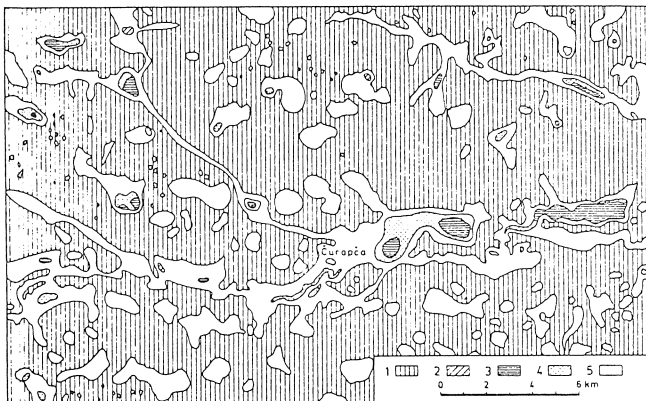
図-7 火星の表面地形とアラスの比較 A : マリーナの映像による火星の表面地形 B : ヤクーツク地方中央部のアラス
