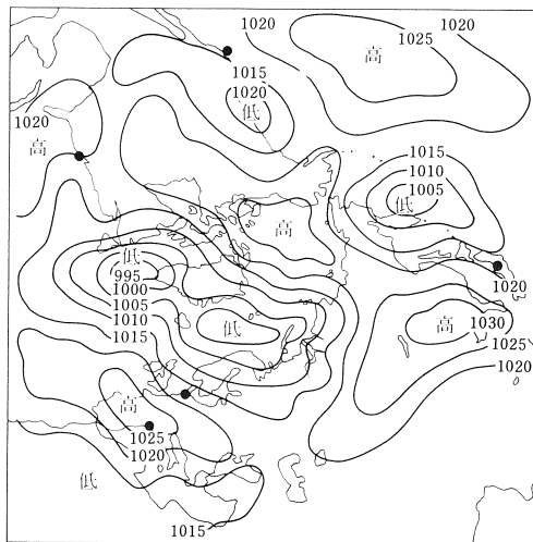
C型の平均地上気圧図
