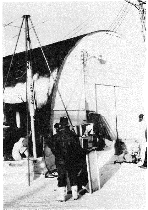
写真—1 第15次用サーモドリル（プロトタイプ）のテスト（1973年10月）
