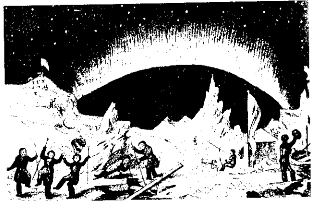
図-6 ロス隊がプーシヤ半島で北磁極点を発見した時の模様
