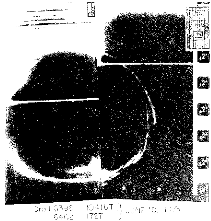
図-1 人工衛星 DMSP によって写された南極大陸上に現われたオーロラで、オーロラ・オーヴァルと呼ばれ環状に分布しているのがわかる。
